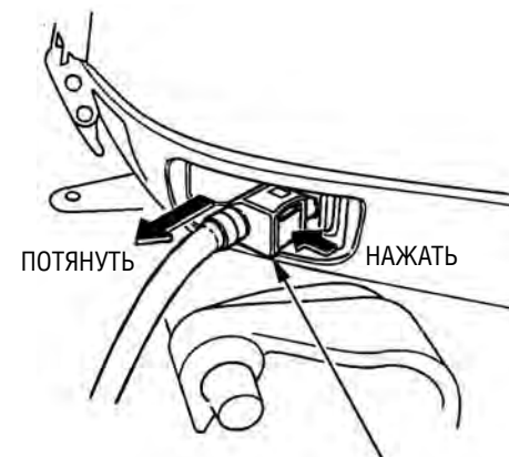
ШТУЦЕР ДЛЯ ПРИСОЕДИНЕНИЯ ТОПЛИВОПРОВОДА
