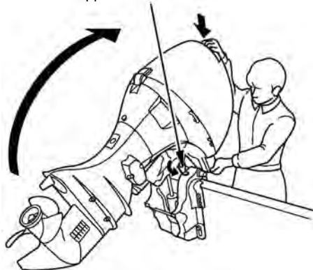
РЫЧАГ ФИКСАТОРА МОТОРА В ПОДНЯТОМ ПОЛОЖЕНИИ
